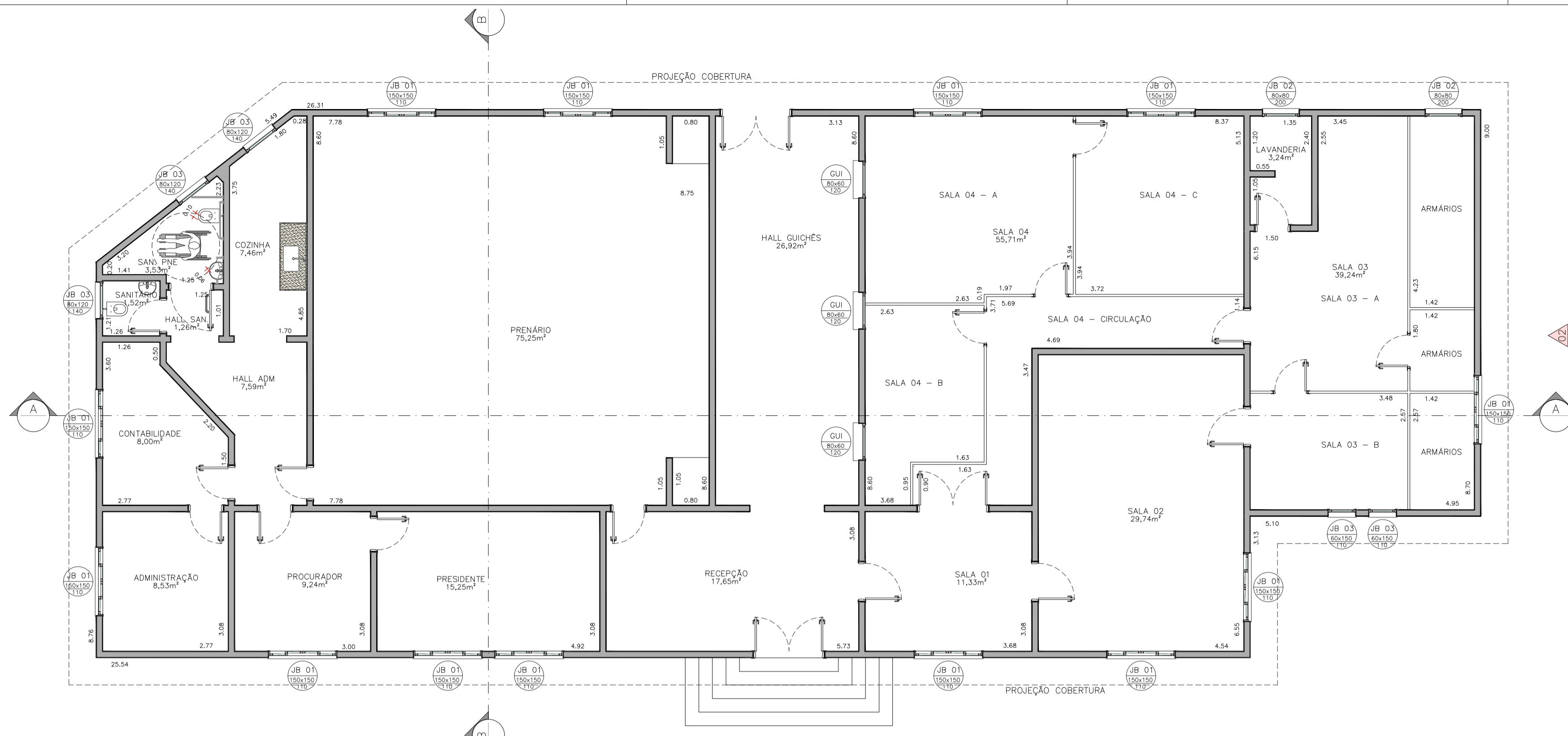
PLANTA BAIXA – CONDIÇÃO PROJETADA ESC. 1:75
